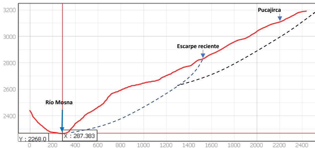
Figura 4. Perfil longitudinal, muestra la morfología ondulada, ladera arriba, desde el río Puchca hasta el caserío Pucajirca, donde se aprecia el salto del deslizamiento reactivado.
