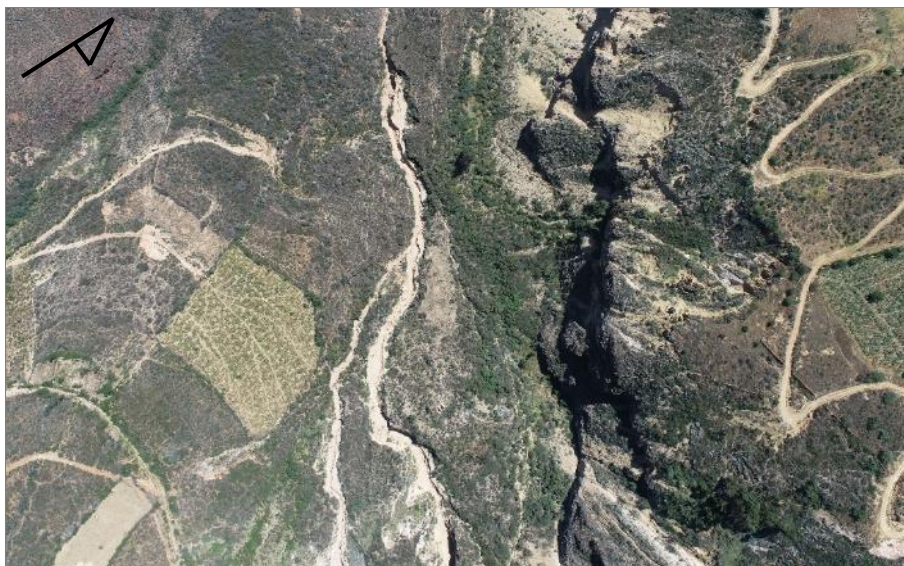
Fotografía 1. Vista de erosión de ladera en cárcavas, con pendientes fuertes a muy fuertes, así también se observa pendientes abruptas hacia el noreste.
