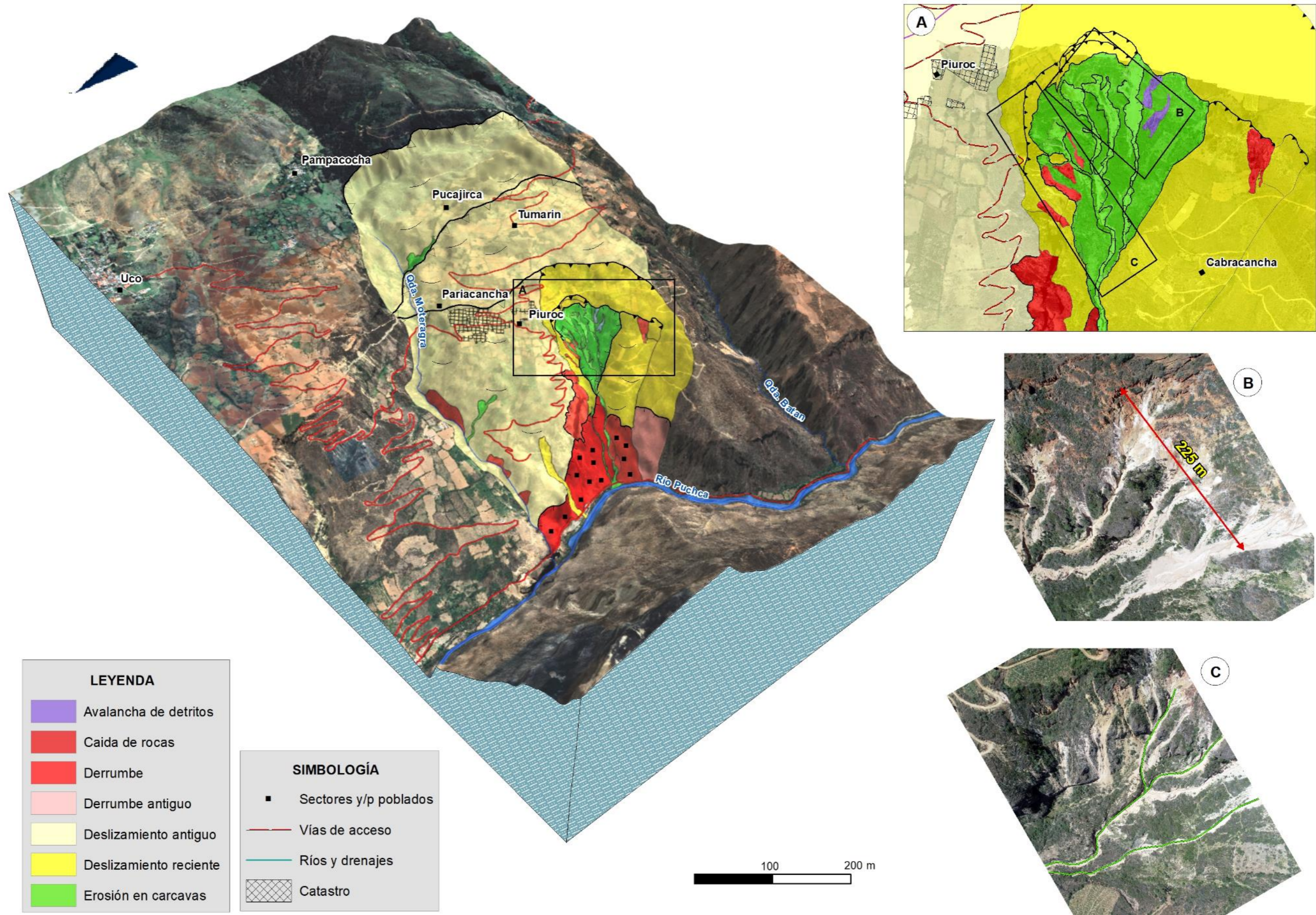
Figura 8. Peligros geológicos por movimientos en masa y otros peligros geológicos identificados en el centro poblado de Pariacancha.
