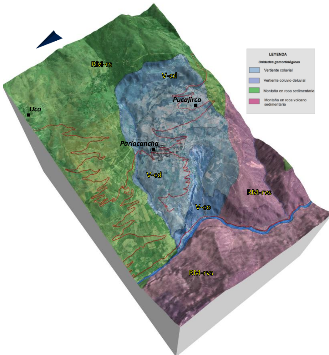
Figura 5. Sub unidades geomorfológicas identificadas en el centro poblado de Pariacancha. RM-rs: Montaña modelada en roca sedimentaria, RM-rvs: Montaña modelada en rocas vulcano-sedimentarias, V-cd: Vertiente coluvio deluvial y V-co: Vertiente coluvial.
