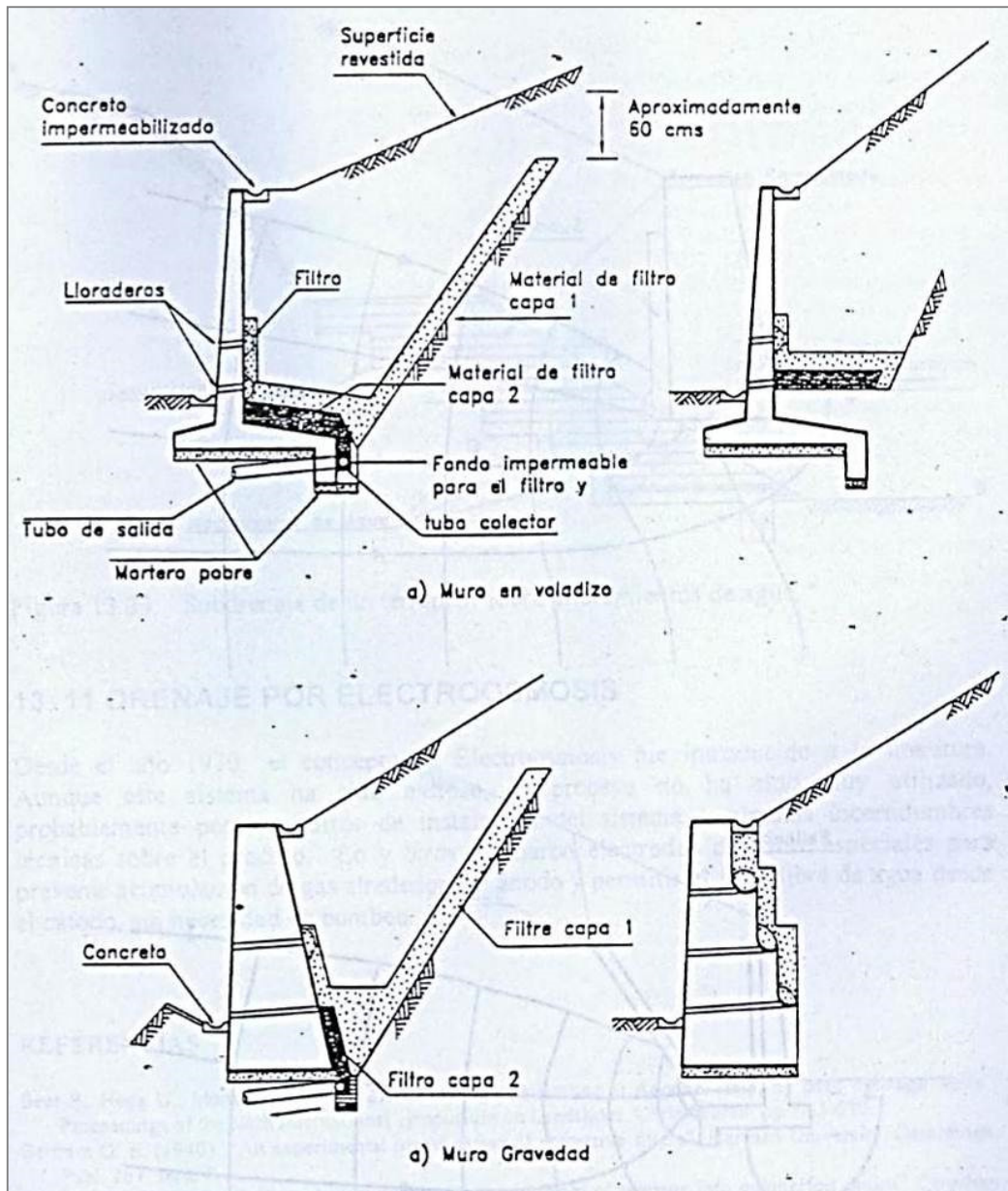
Figura 32: Ejemplos de subdrenajes con muros de contención.
