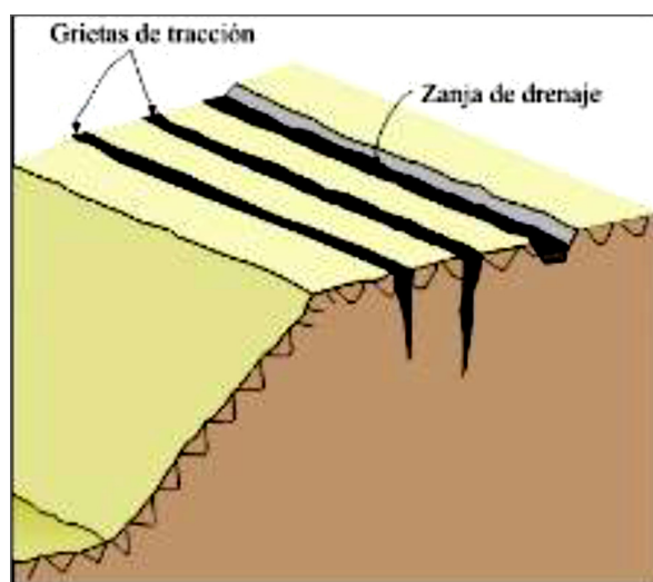
Figura 24: Disposición de zanjas en un talud (Tomado de INGEMMET, 2000)
