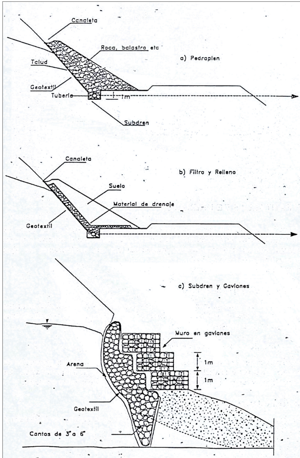
Figura 31: Ejemplos de subdrenes de pantalla
