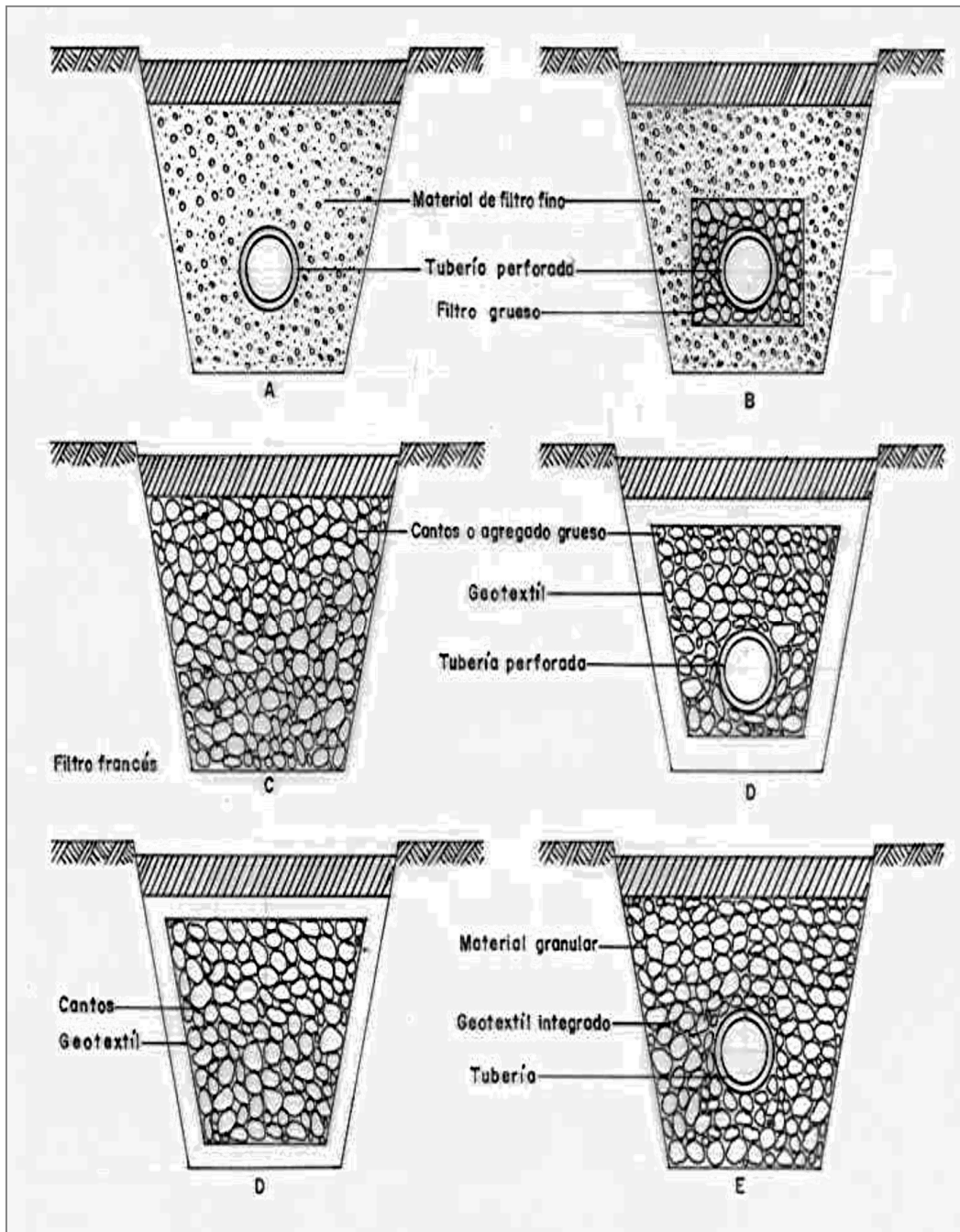
Figura 25: Tipos de subdrenes interceptores (Adaptado de Suárez, 1998)
