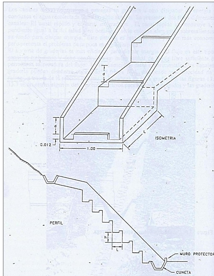
Figura 23: Canal de entrega con gradas de disipación.
