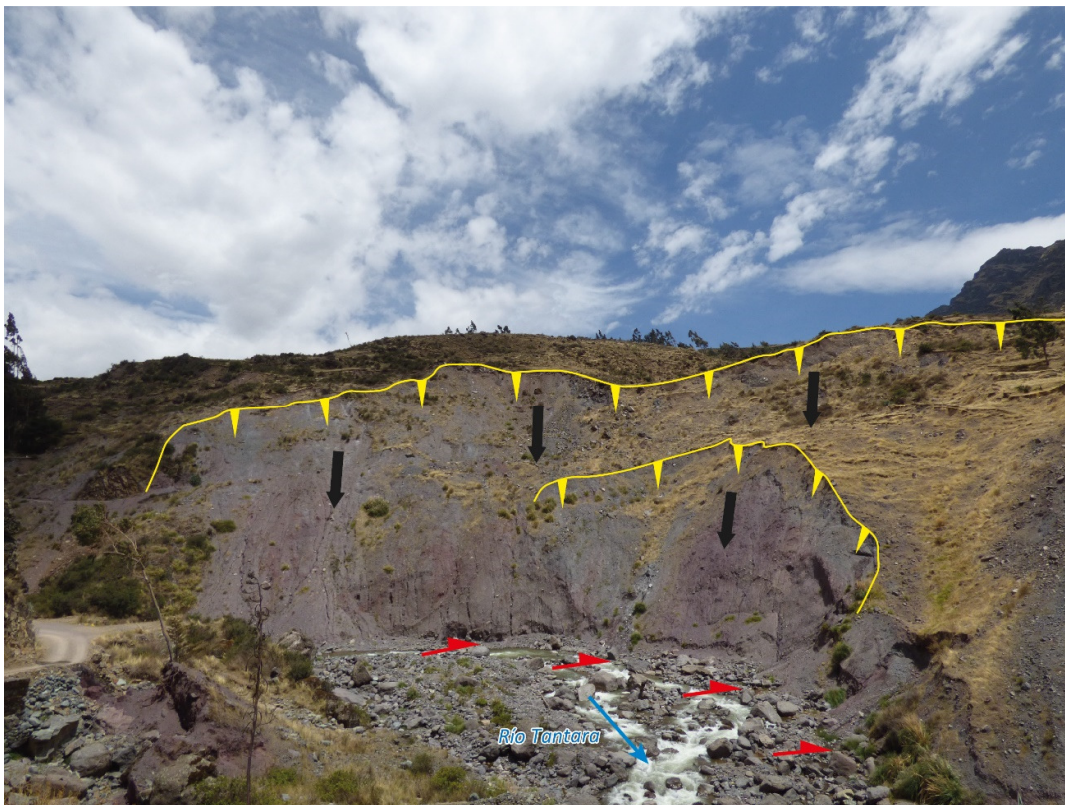
Figura 14. Derrumbes al pie del deslizamiento (líneas amarillas) reactivados debido a la acción erosiva del río Tantara (flechas rojas) que viene socavando la base del talud.
