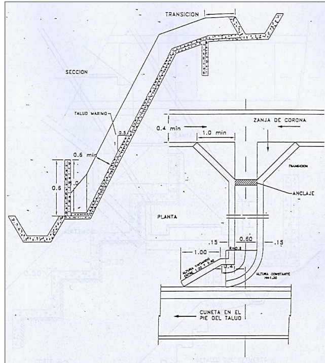
Figura 22: Detalle de un canal rápido de entrega
