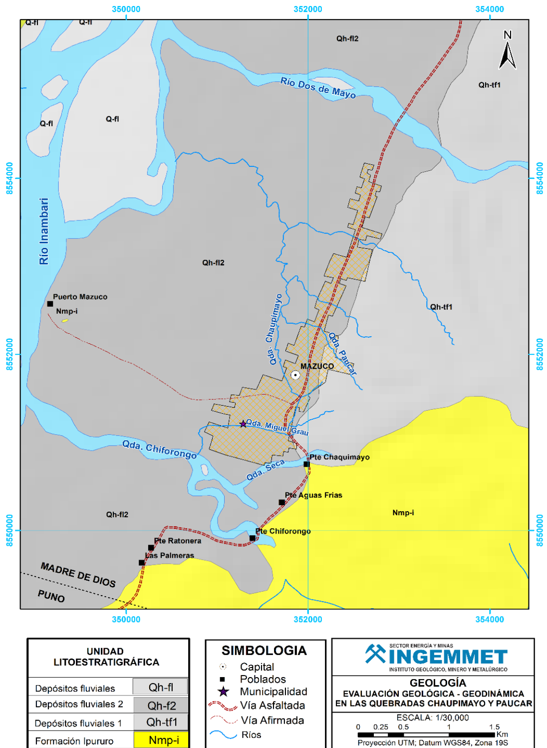
Figura 3. Mapa geológico de la zona de estudio. Tomado del mapa geológico del cuadrángulo de Mazuco -27v4 (Ingemmet, 2015).
