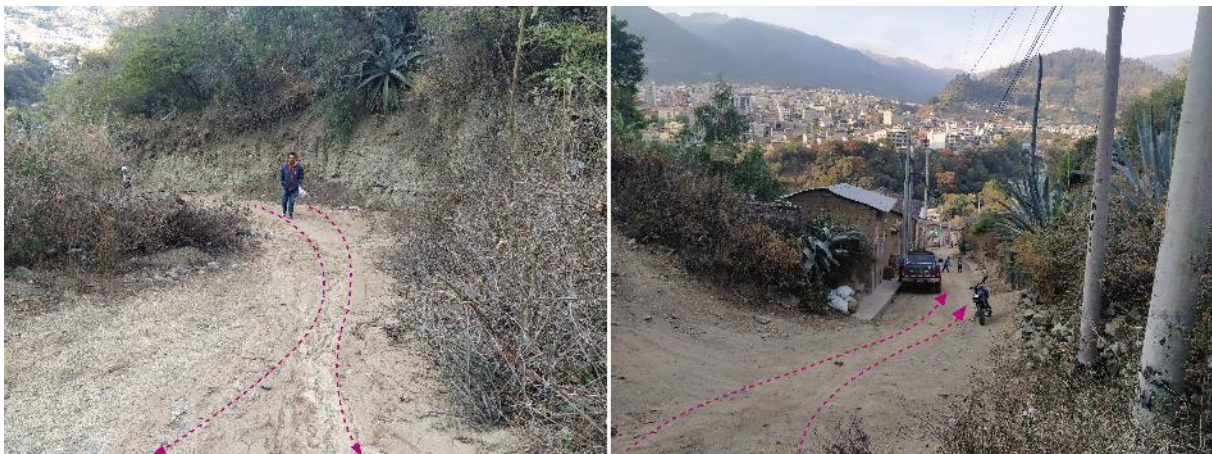
Figura 19. Evidencia de flujo de lodos en el Barrio Mariño, desembocadura de la quebrada Anishuayjo
