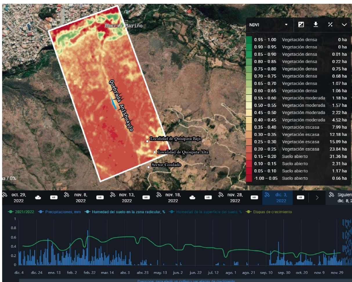
Figura 5. Visualización de los datos meteorológicos del sistema Crop Monitoring, muestra que el 2022, los índices de vegetación en la quebrada Anishuayjo corresponden a vegetaciones escasas y moderadas.
