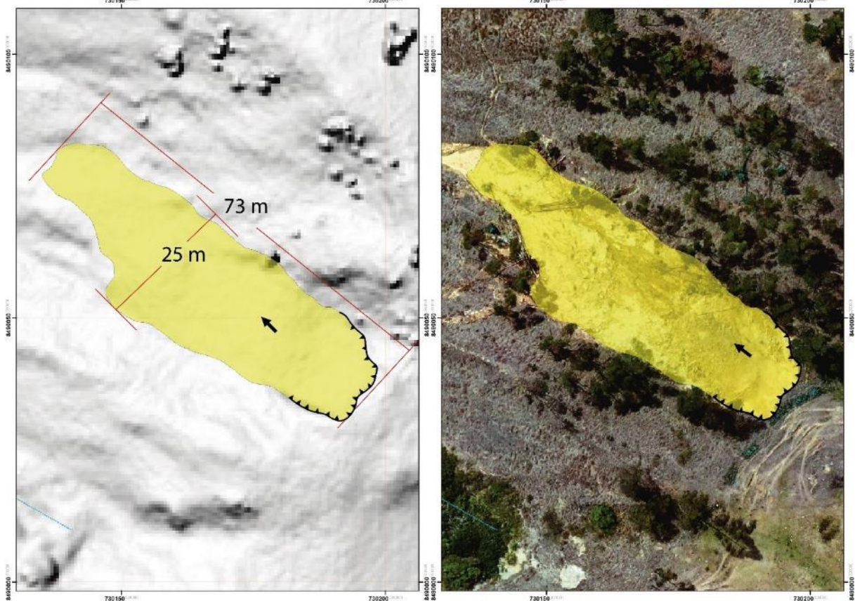
Figura 17 Dimensiones de deslizamiento de Quisipata Baja.
