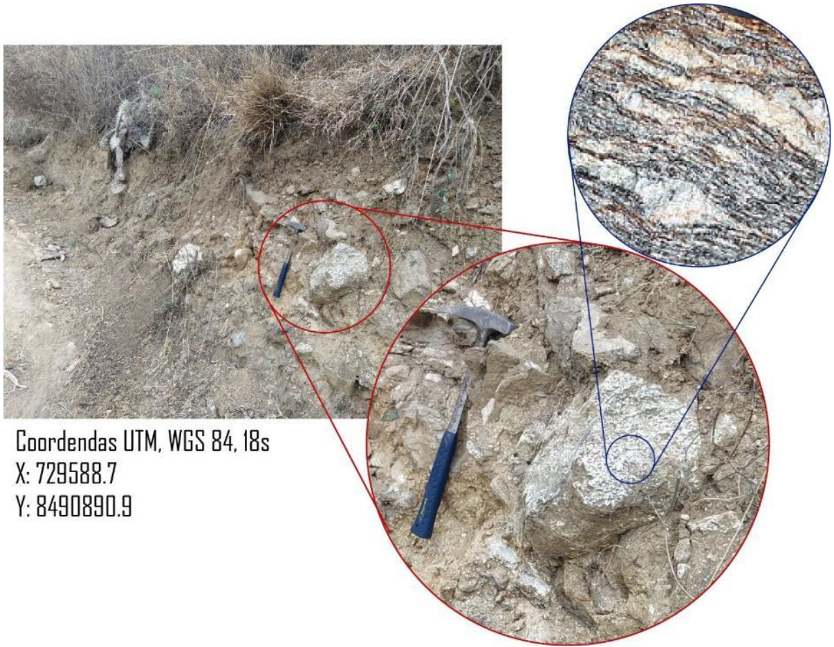
Figura 8. Ortogneis en la parte baja de la quebrada Anishuayjo, se muestra la roca fragmentada.
