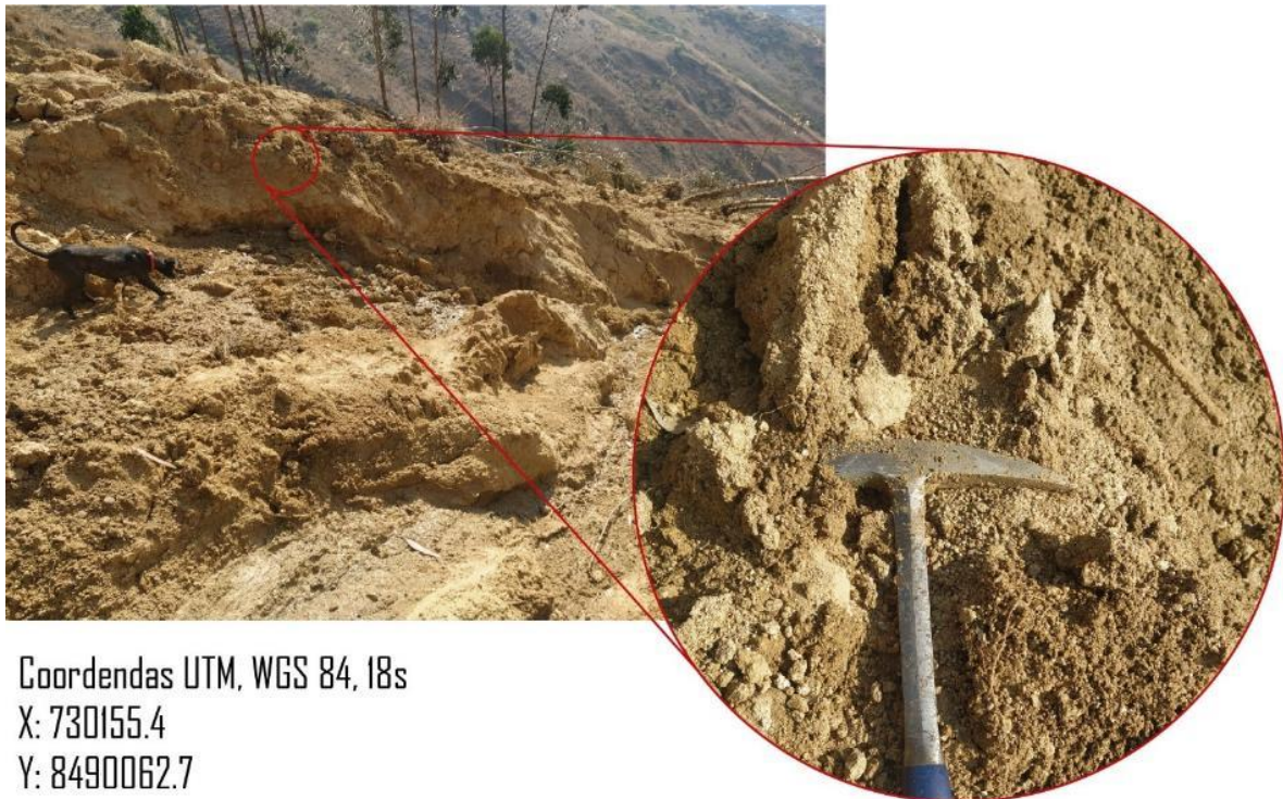
Figura 9. Ortogneis en la parte alta de la quebrada Anishuayjo, se muestra la roca altamente meteorizada.
