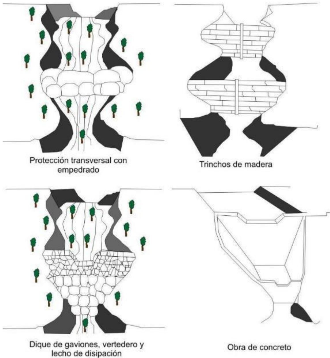
Figura 24. Obras hidráulicas transversales para el control de erosión en cárcavas.
