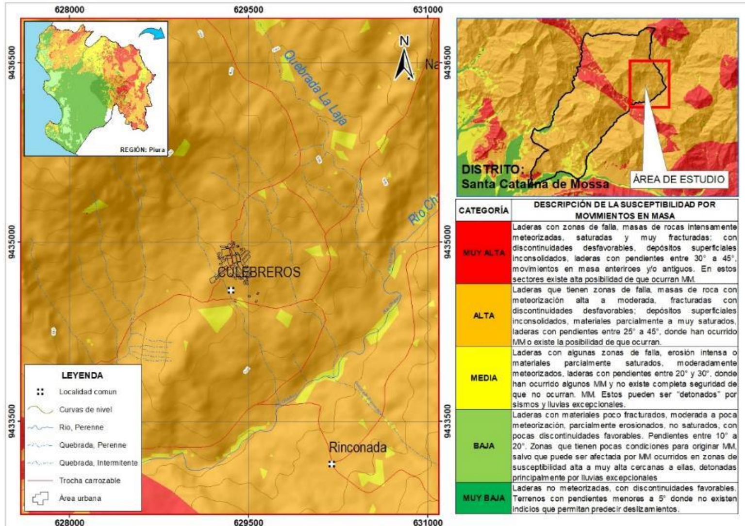
Figura 1. Mapa de susceptibilidad a movimientos en masa a escala 1:100 000 de la zona de evaluación (Vilchez et al., 2017).
