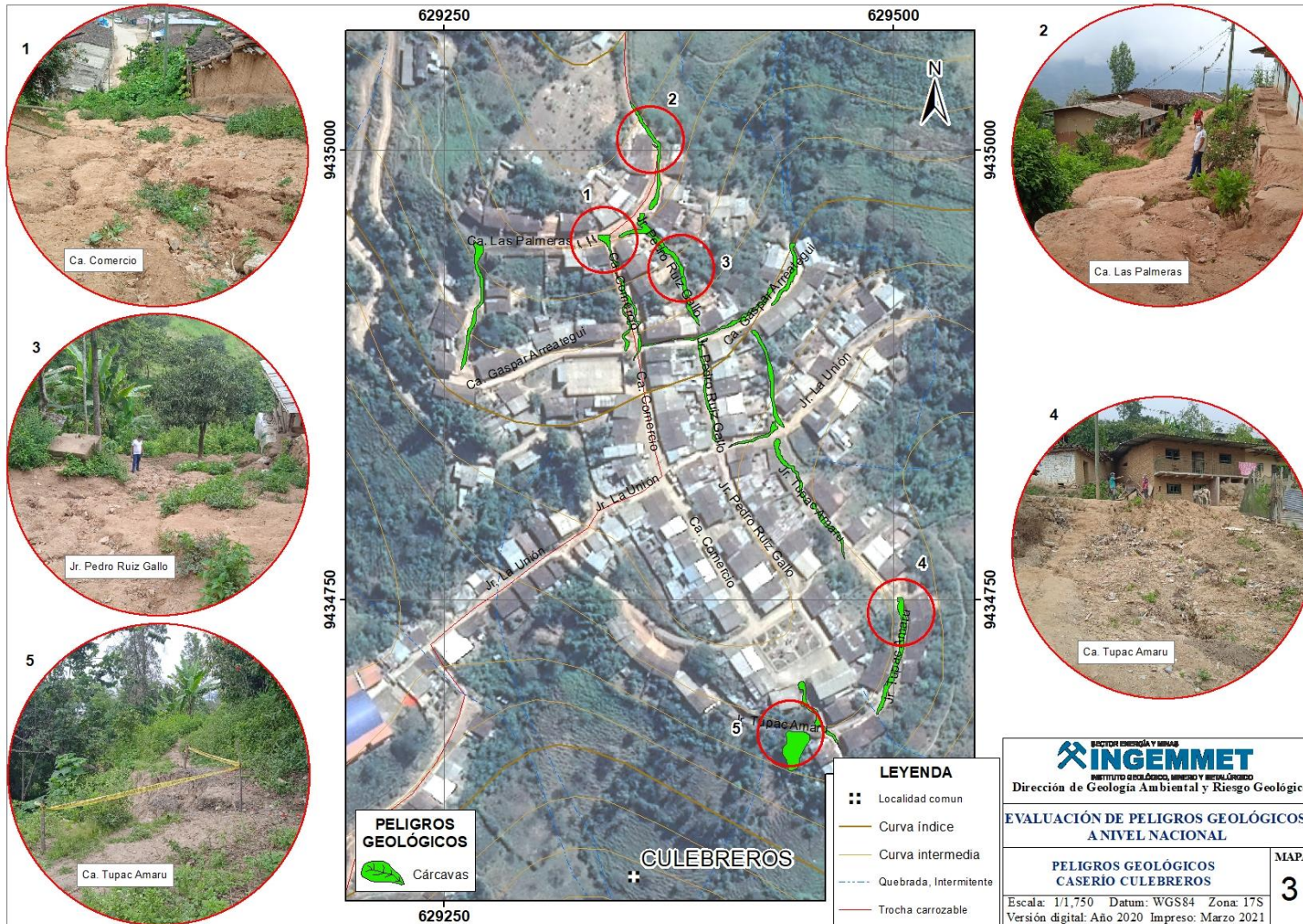
Mapa 3. Peligros geológicos del área evaluada.
