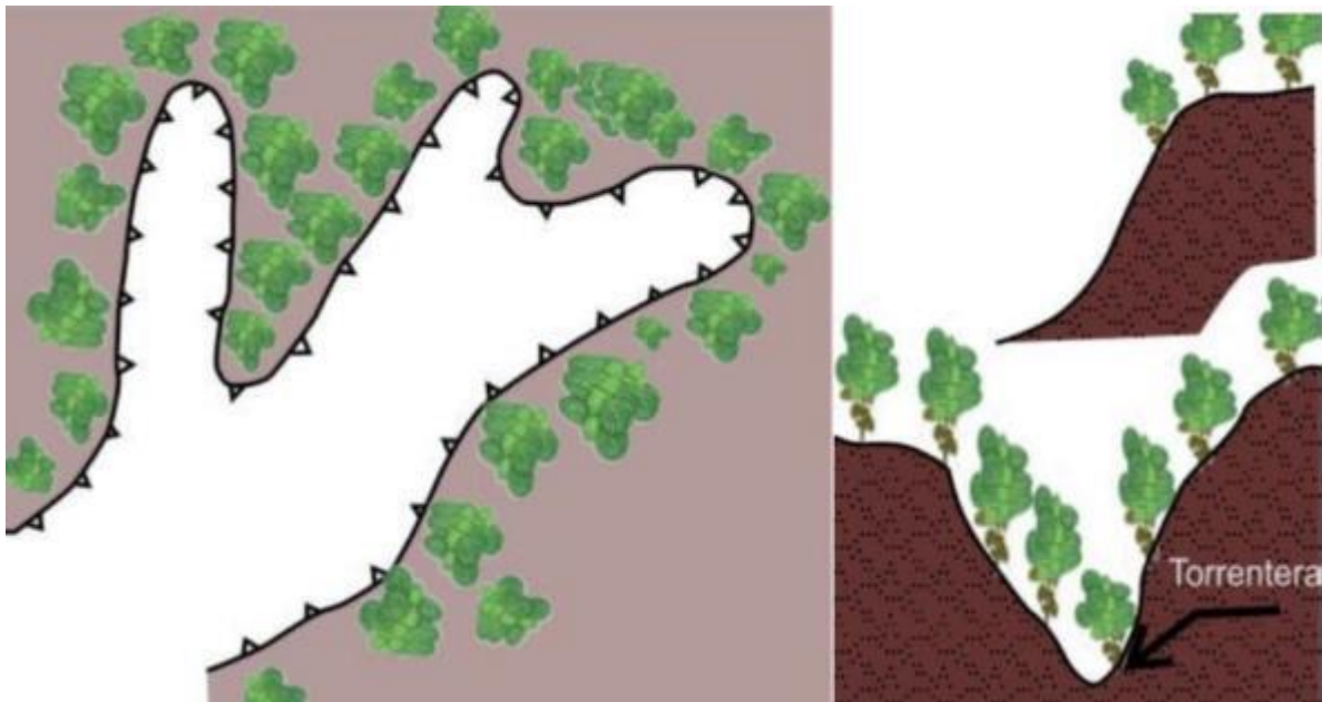
Figura 23. Vista en planta y perfil de los procesos de forestación en cabeceras y márgenes de las áreas inestables.
