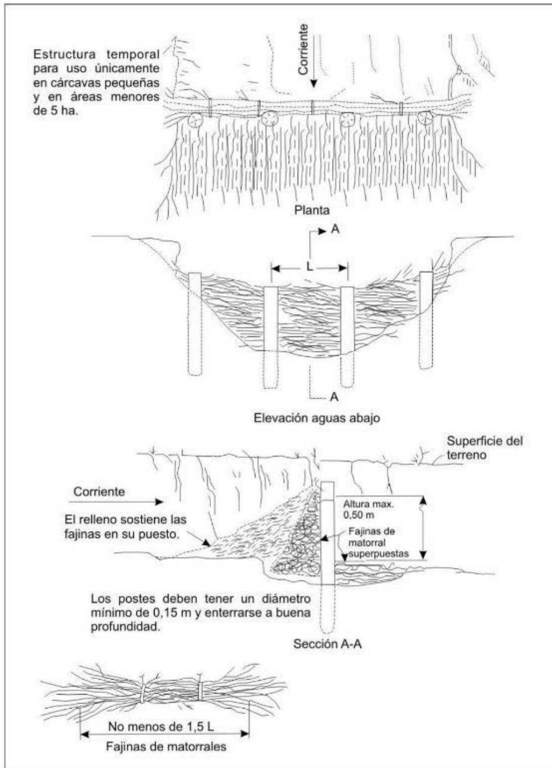
Figura 26. Presas de matorral tipo una hilera de postes (adaptado de Valderrama et al., 1964).
