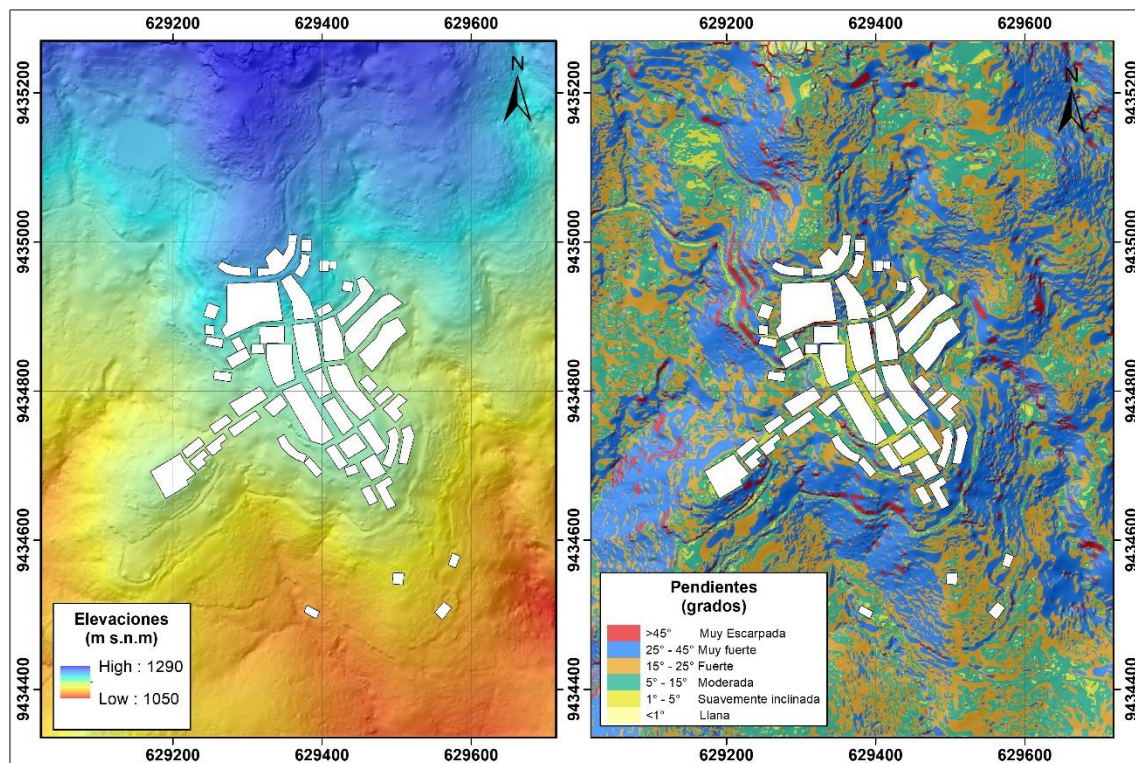
Figura 4. Elevaciones y rangos de pendientes en el área de evaluación.
