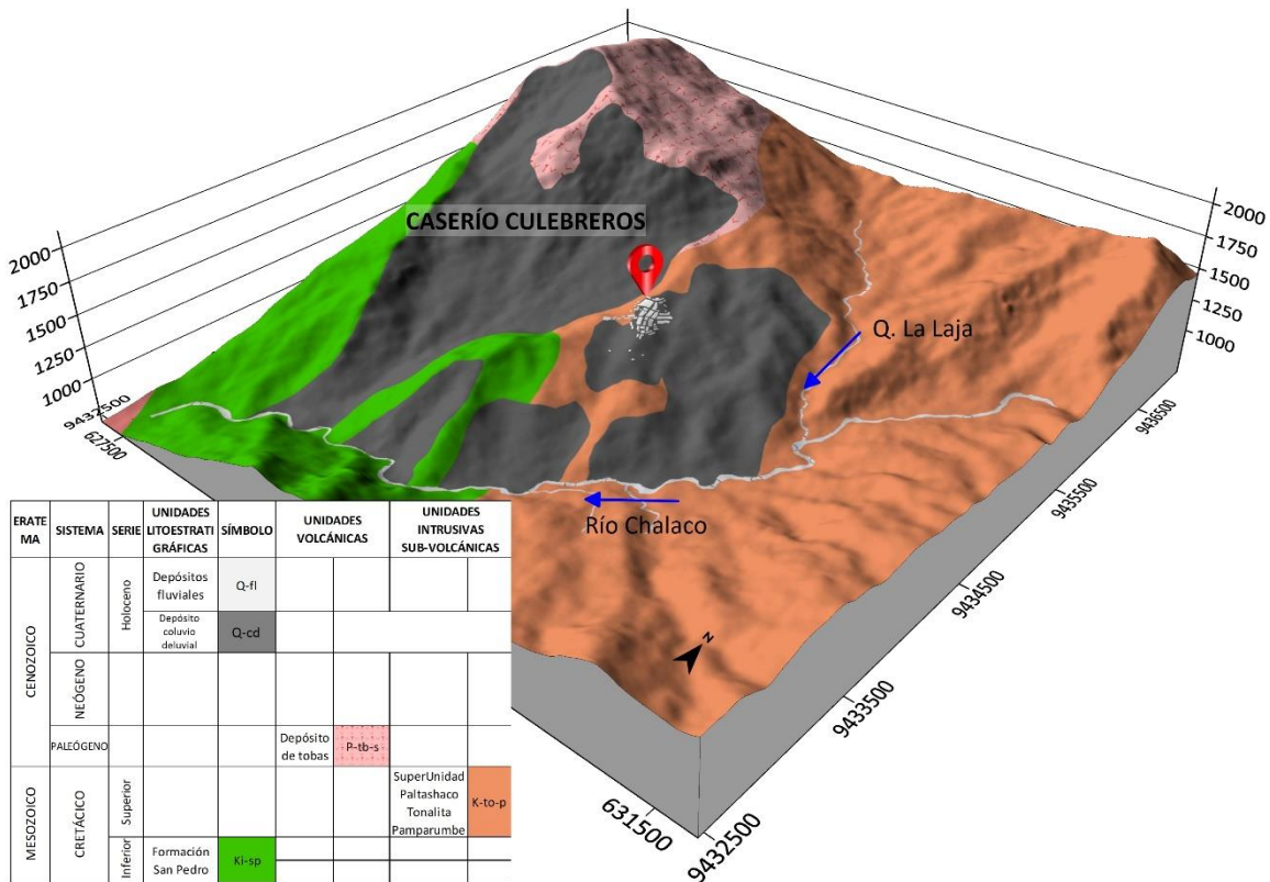
Figura 3. Unidades litoestratigráficas en el caserío Culebreros.
