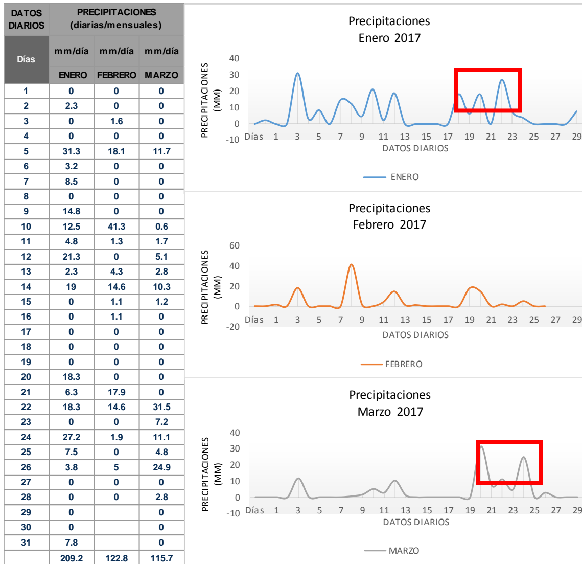
Cuadro 6. Datos de precipitación mensual enero – marzo 2017.
