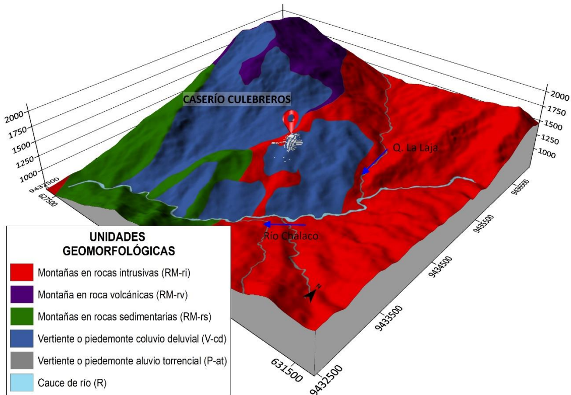
Figura 8. Unidades geomorfológicas en el caserío Culebreros.
