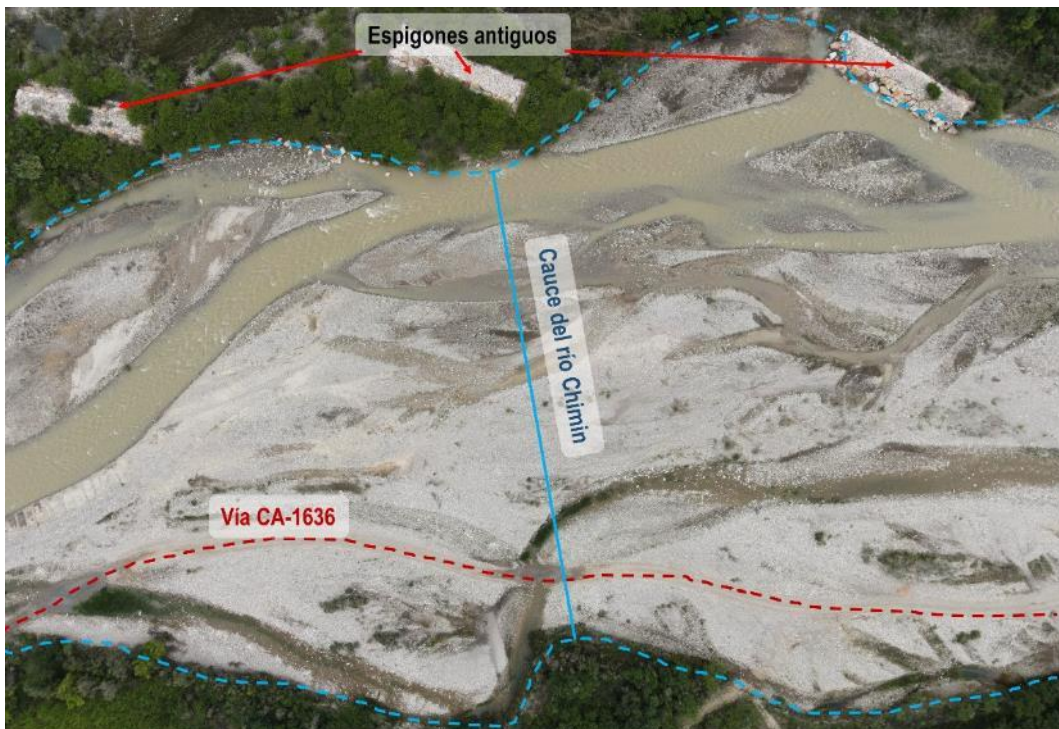
Figura 7. Vista del cauce del río Chimin por donde cruza un tramo de la vía vecinal CA-1636.
