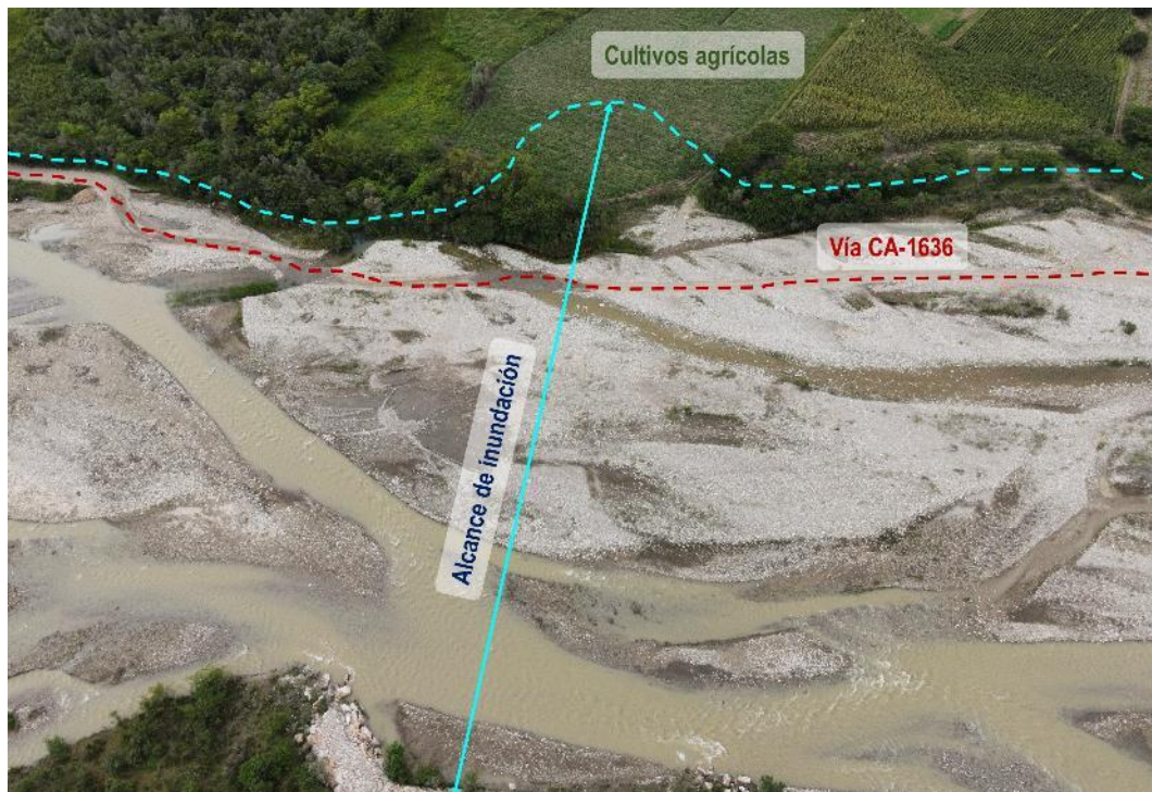
Figura 12. Lugar del perfil A-A', donde se aprecia a la vía vecinal CA-1636 y cultivos susceptibles a inundación fluvial. Ubicación: E: 811130, N: 9166622.
