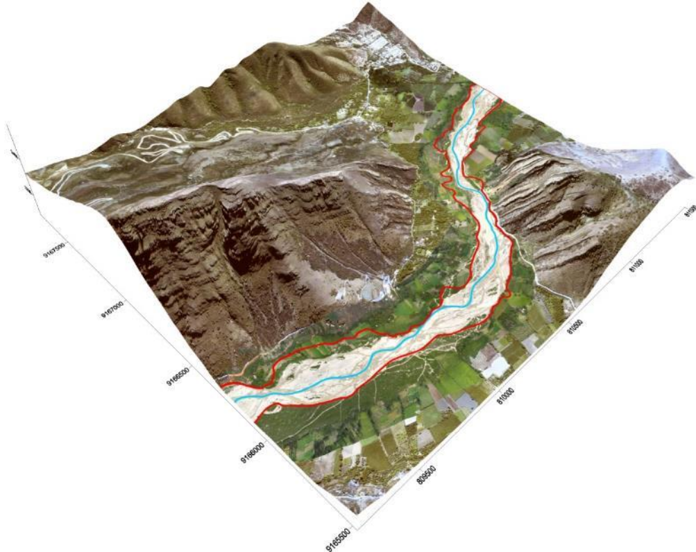
Figura 8. Modelo 3D del valle del río Chimin, mostrando el curso principal en celeste y el límite de inundación fluvial en rojo.
