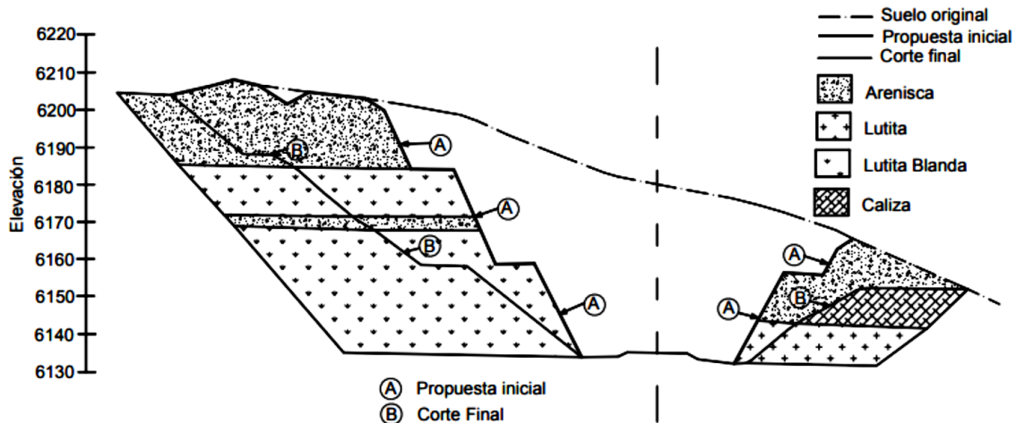
Figura 26. Talud con ángulo uniforme y talud con excavado de forma escalonada con bermas y bancos (Gonzáles, 2002).
