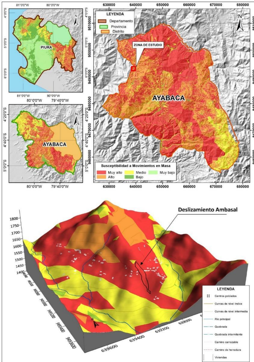
Figura 1. Mapa de susceptibilidad a movimientos en masa a escala 1:250 000 de la zona de evaluación (Vílchez, 2013).
