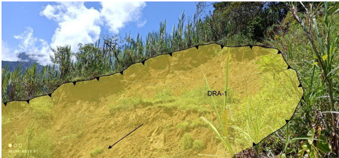
Figura 15. Escarpe visto desde el flanco izquierdo del deslizamiento.
