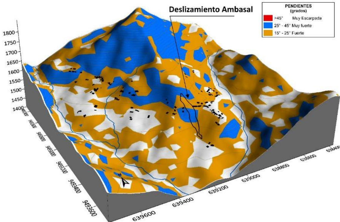
Figura 23. Rangos de pendientes que condicionan la ocurrencia de movimientos en masa.
