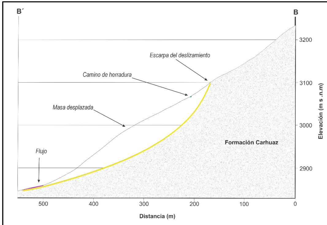
Figura 26. Esquema de sección del deslizamiento de la localidad de Shauri.
