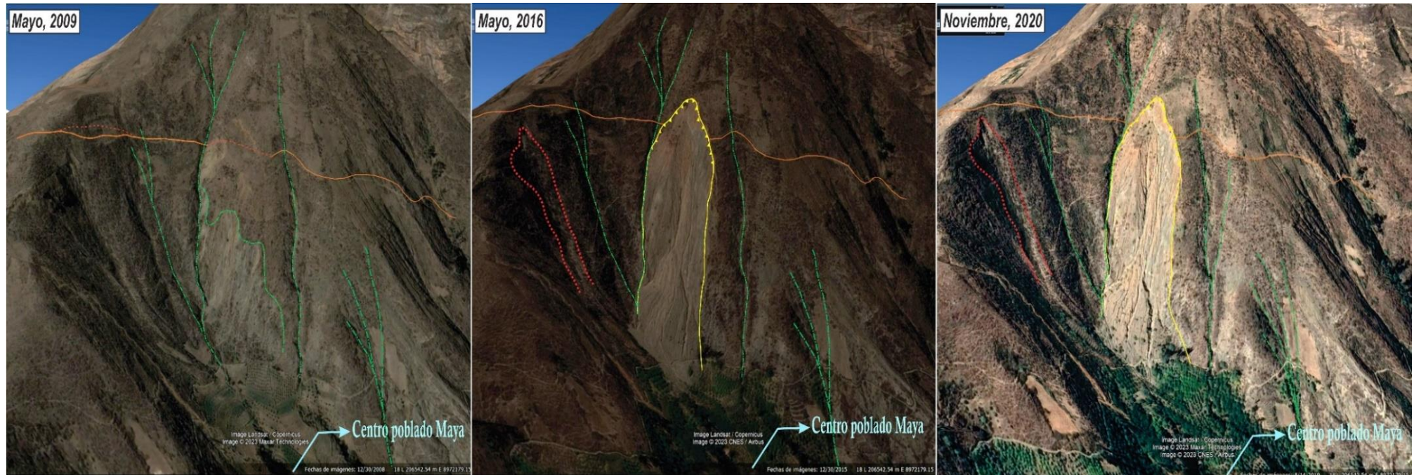
Figura 22. Análisis multitemporal que muestra la evolución del deslizamiento de la localidad de Shauri, usando imágenes de la plataforma de Google Earth e imágenes tomadas del dron tomadas el 2022.
