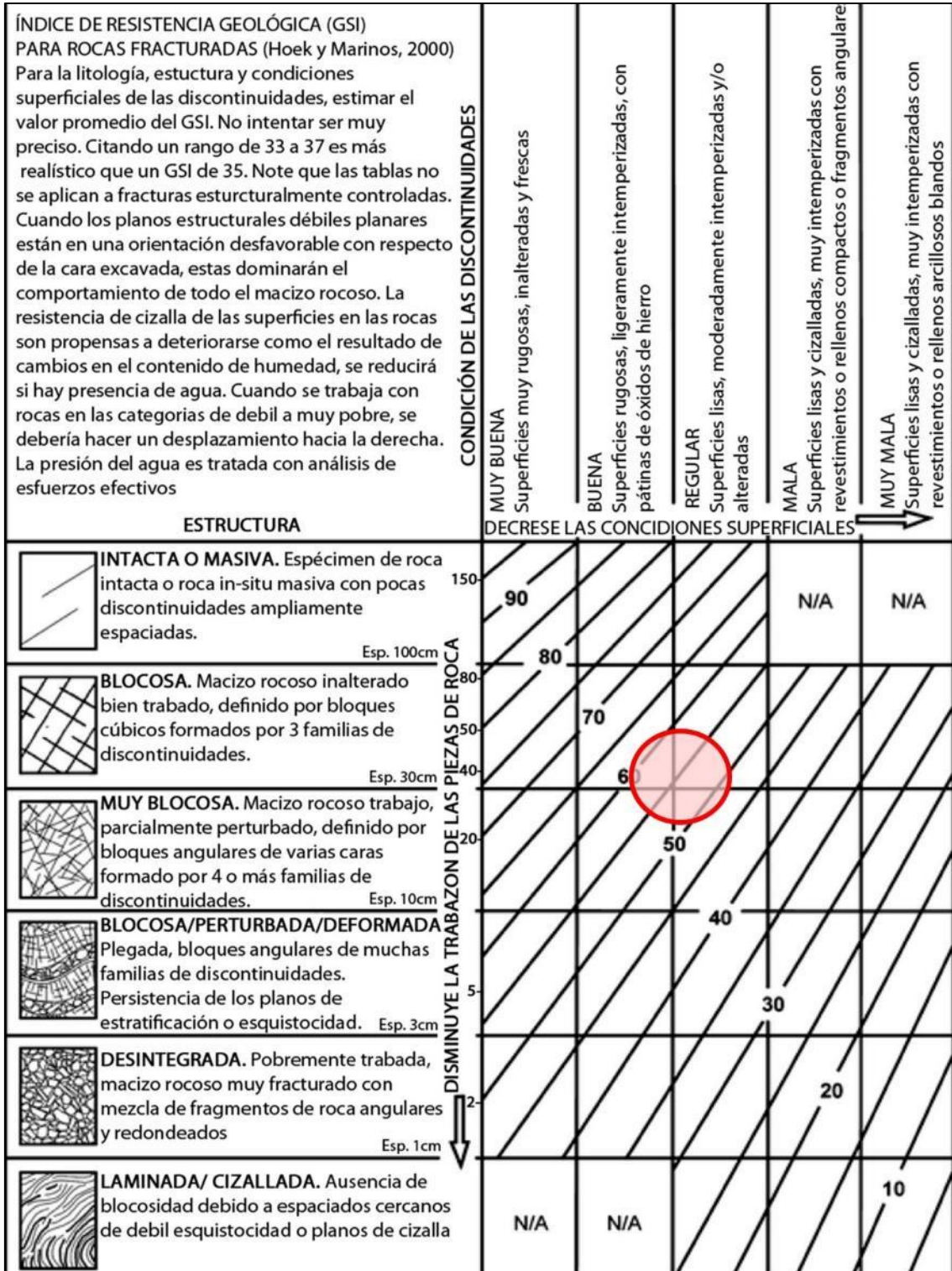
Figura 4. Estructura y calidad de las discontinuidades del macizo rocoso del Plutón Rushos, GSI promedio de entre 50 a 60. Fuente: Tabla del Índice Geológico de Resistencia GSI (Hoek, 2007).
