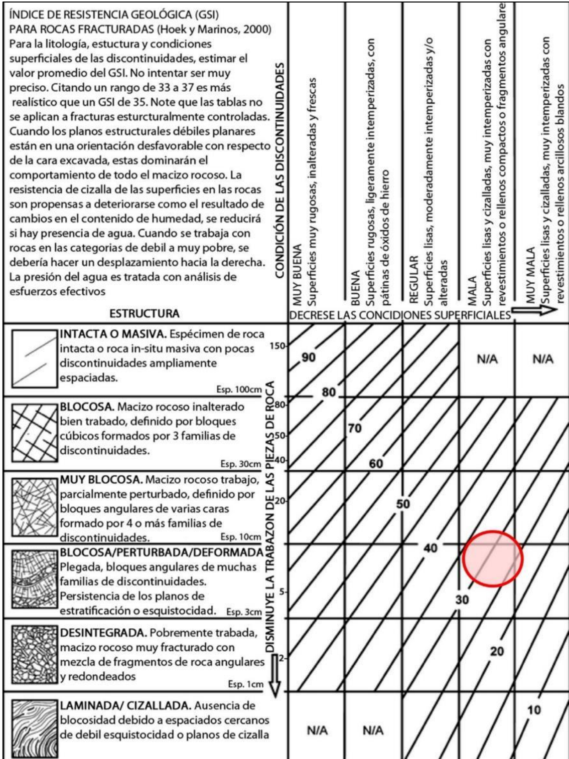
Figura 4. Estructura y calidad de las discontinuidades del macizo rocoso del Grupo Quilquiñán, GSI promedio de entre 25 a 35. Fuente: Tabla del Índice Geológico de Resistencia GSI (Hoek, 2007).
