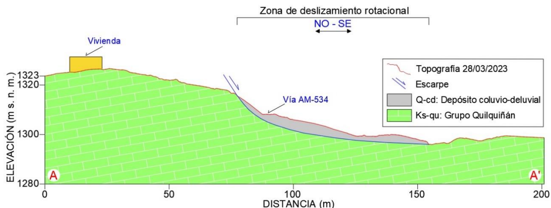
Figura 12. Perfil longitudinal A-A' que representa la distribución de los materiales geológicos, agrietamientos y estructuras expuestas a daños.
