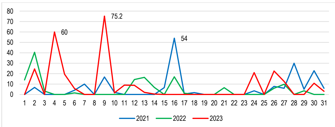
Figura 3. Precipitación diaria del mes de marzo entre los años 2021-2023, en la Estación Aramango (Provincia Bagua). Fuente: Senamhi.
