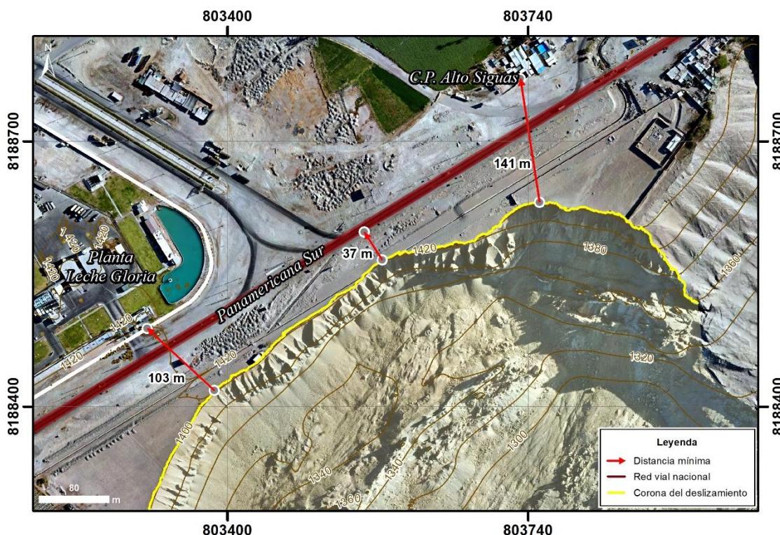
Figura 8. Medición de distancias mínimas realizadas sobre ortomosaico de noviembre de 2022, entre el límite de la parte superior del deslizamiento (corona) e infraestructura crítica (Carretera Panamericana Sur, Planta de leche Gloria y centro poblado de Alto Sigüas).
