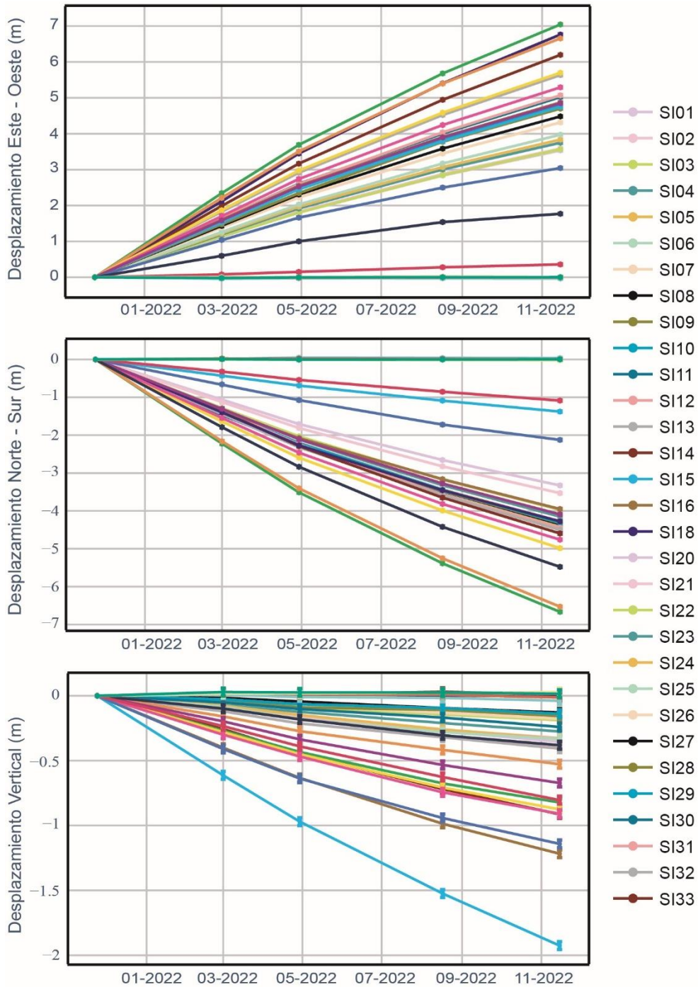
Figura 5. Series temporales de desplazamiento acumulado de las componentes norte-sur, este-oeste y vertical de los puntos de control instalados en el área de estudio. Las series temporales se graficaron a partir de la data obtenida en las cinco campañas de medición, entre noviembre de 2021 y noviembre de 2022.
