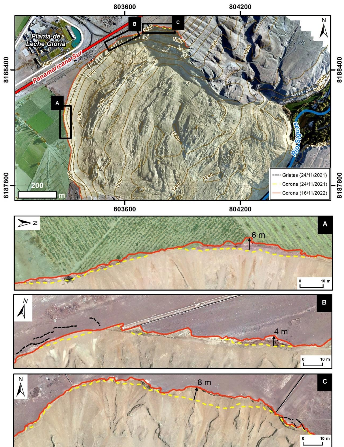
Figura 6. Mapa de comparación multitemporal del avance retrogresivo de la corona del deslizamiento de Sigüas, en las fechas del 24 de noviembre de 2021 y 16 de noviembre de 2022. Los detalles A, B y C muestran la retrogresión máxima aproximada en cada sector.
