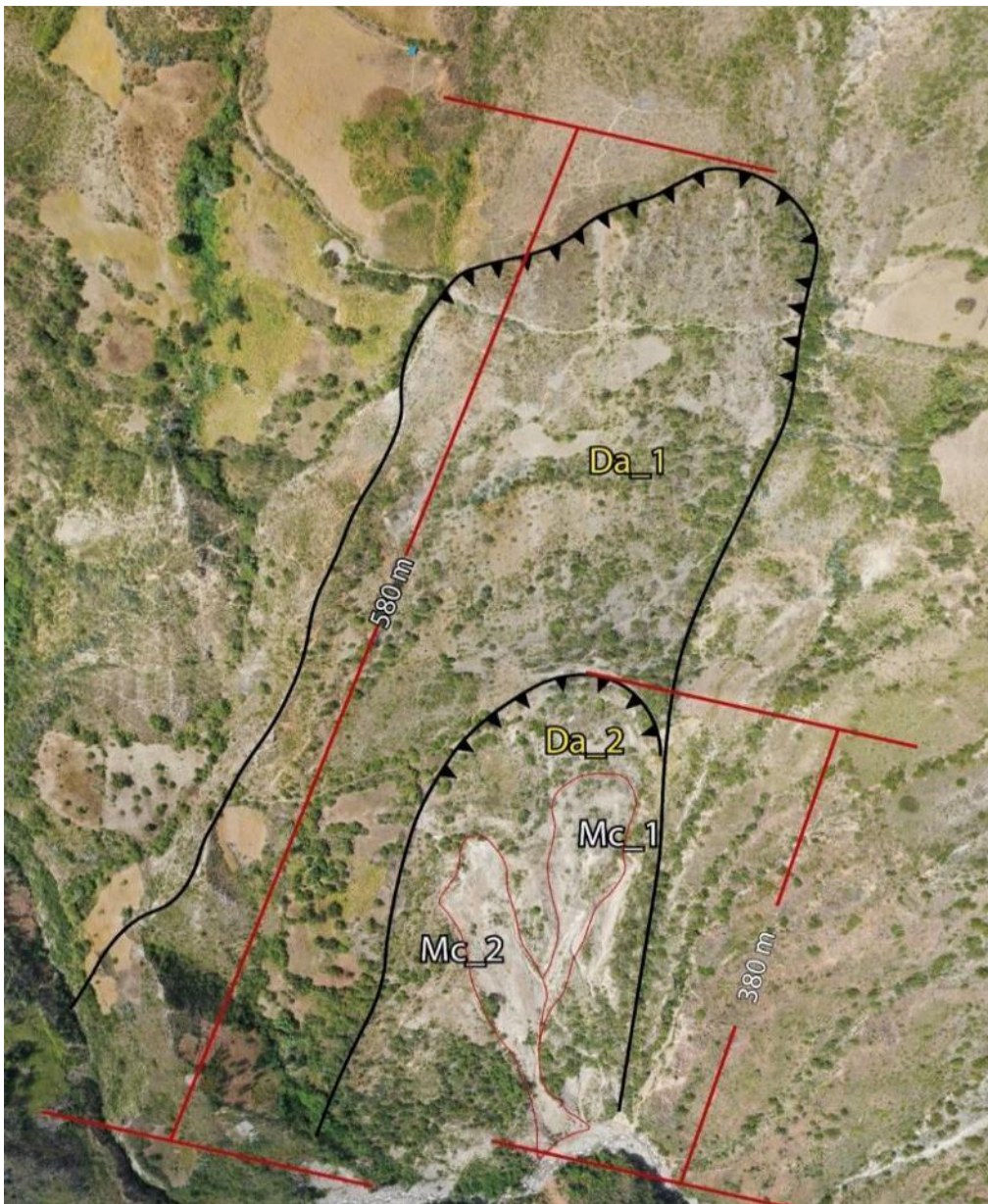
Figura 10. Muestra los deslizamientos activos Da_1 y Da_2, ubicados longitudinalmente a 465 m lineales del C.P Pueblo Libre y a una diferencia de alturas de 174 m entre el poblado y la corona principal.
