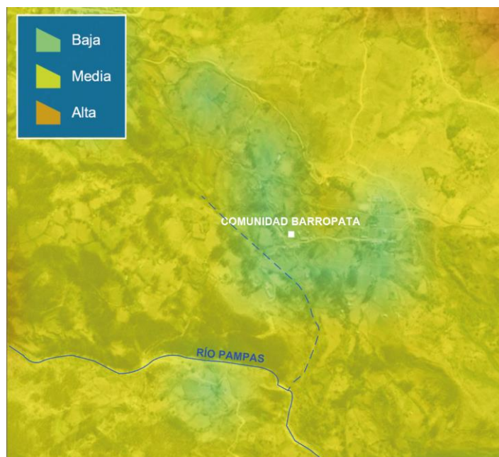
Figura 1: El sector de Barropata, se encuentra en una zona de Susceptibilidad media a baja a movimientos en masa (Vilchez M. 2017)
