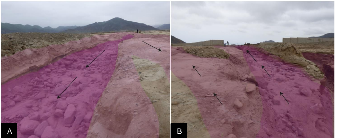
Figura 14. A y B Muestran el flujo de marzo del 2023, se desbordó a la altura del centro poblado Santa Rosa, el flujo recorrió el cauce (violeta) y parte de este fluyó hacia la margen izquierda de cauce (rosado). Las flechas indican la dirección del flujo.
