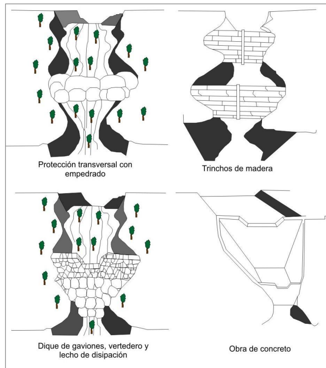
Figura 3. Obras hidráulicas transversales para el control de la erosión en cárcavas, fijación de sedimentos y protección de desaguaderos naturales (Instituto Nacional de Vías, 1998).
