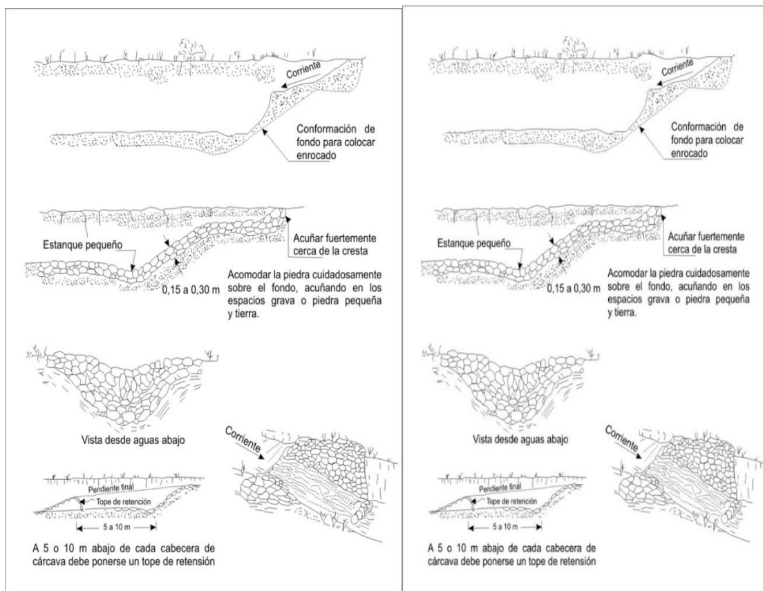
Figura 1. Trincho de piedra para cabecera de cárcava (adaptado de Valderrama et al., 1964).
