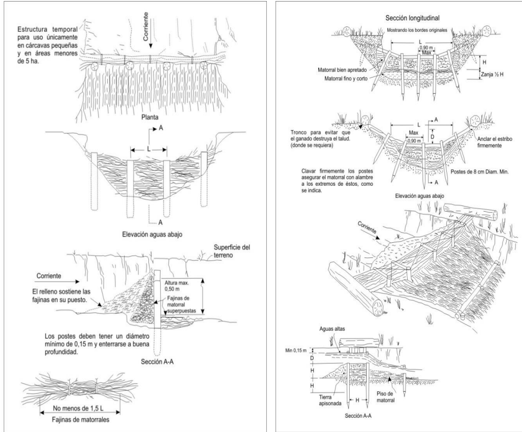
Figura 2. Trincho de matorral tipo una hilera de postes y trincho de matorral tipo doble hilera de postes (adaptado de Valderrama et al., 1964).
